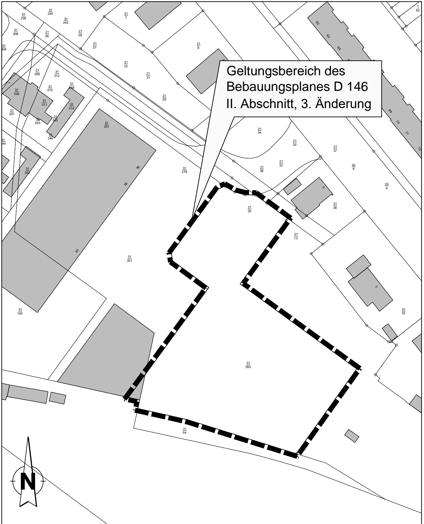
Geltungsbereich des Bebauungsplans D 146 - Abschnitt II, 3. Änderung "Eisenbahndock" M. 1:1.000 FD 361
